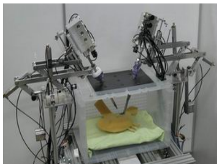
手術ロボット (触覚が手に伝わる)
