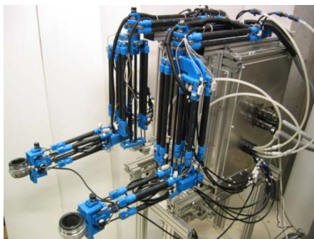
空気圧ゴム人工筋ロボットアーム (柔らかさを持っている)
